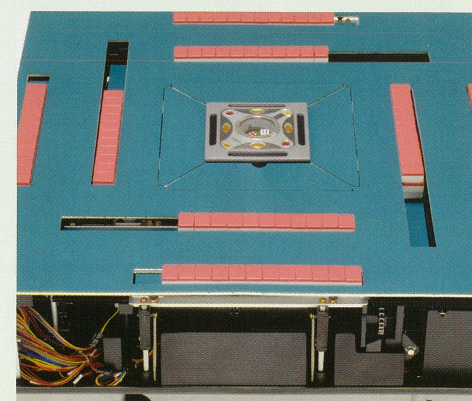
エレベータ上昇途中です。手牌と築牌が同時に天板上に上がります。
