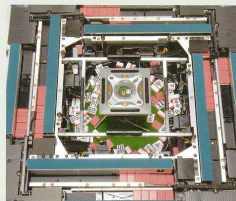
天板を開けた状態です。ホッパー内で牌が攪拌され、4カ所から同時に牌が吸い上げられます。
